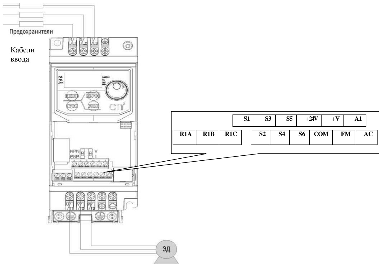
Назначение входных и выходных клемм цепи управления ONI A400
