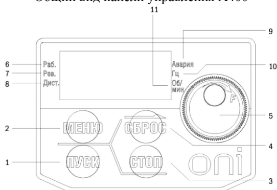
Общий вид панели управления A400
