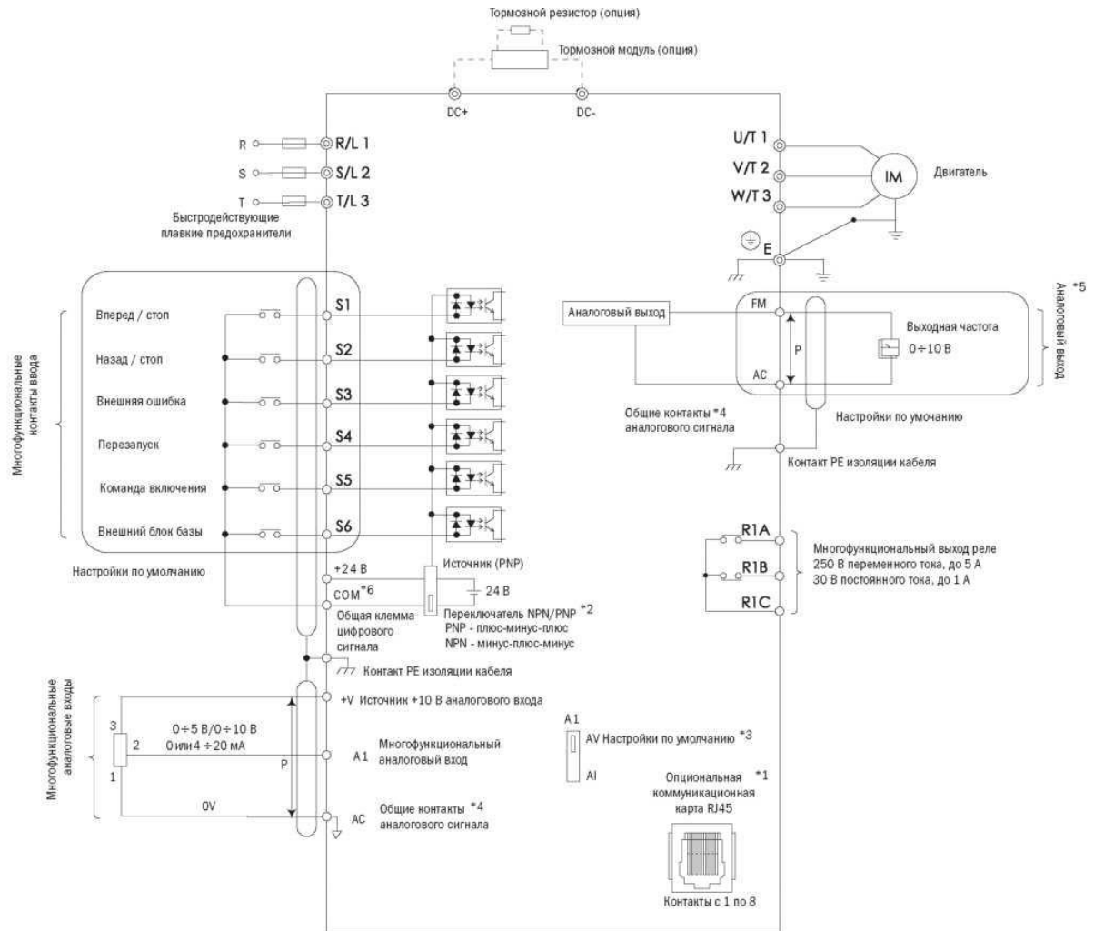
Схема электрических соединений и подключений ONI A400
